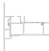
▲スライドレール断面図
