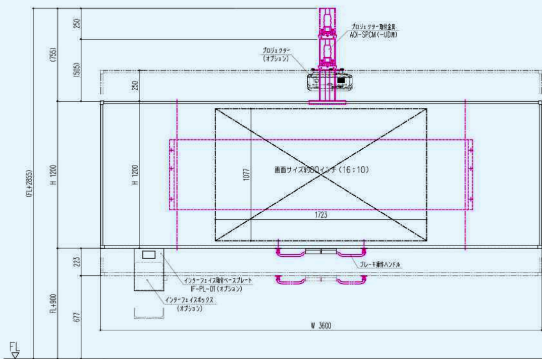
展開図
