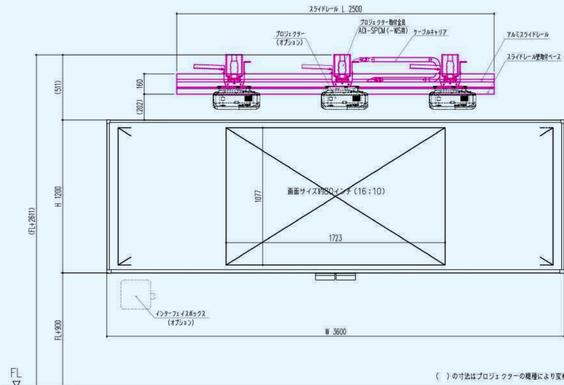
展開図
