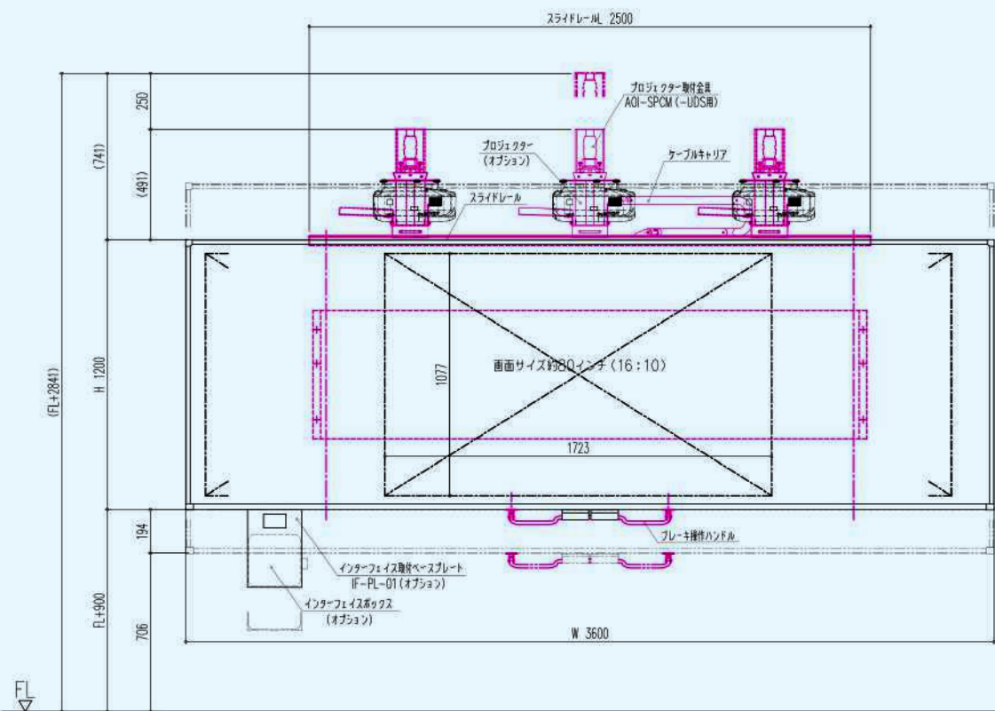
展開図
