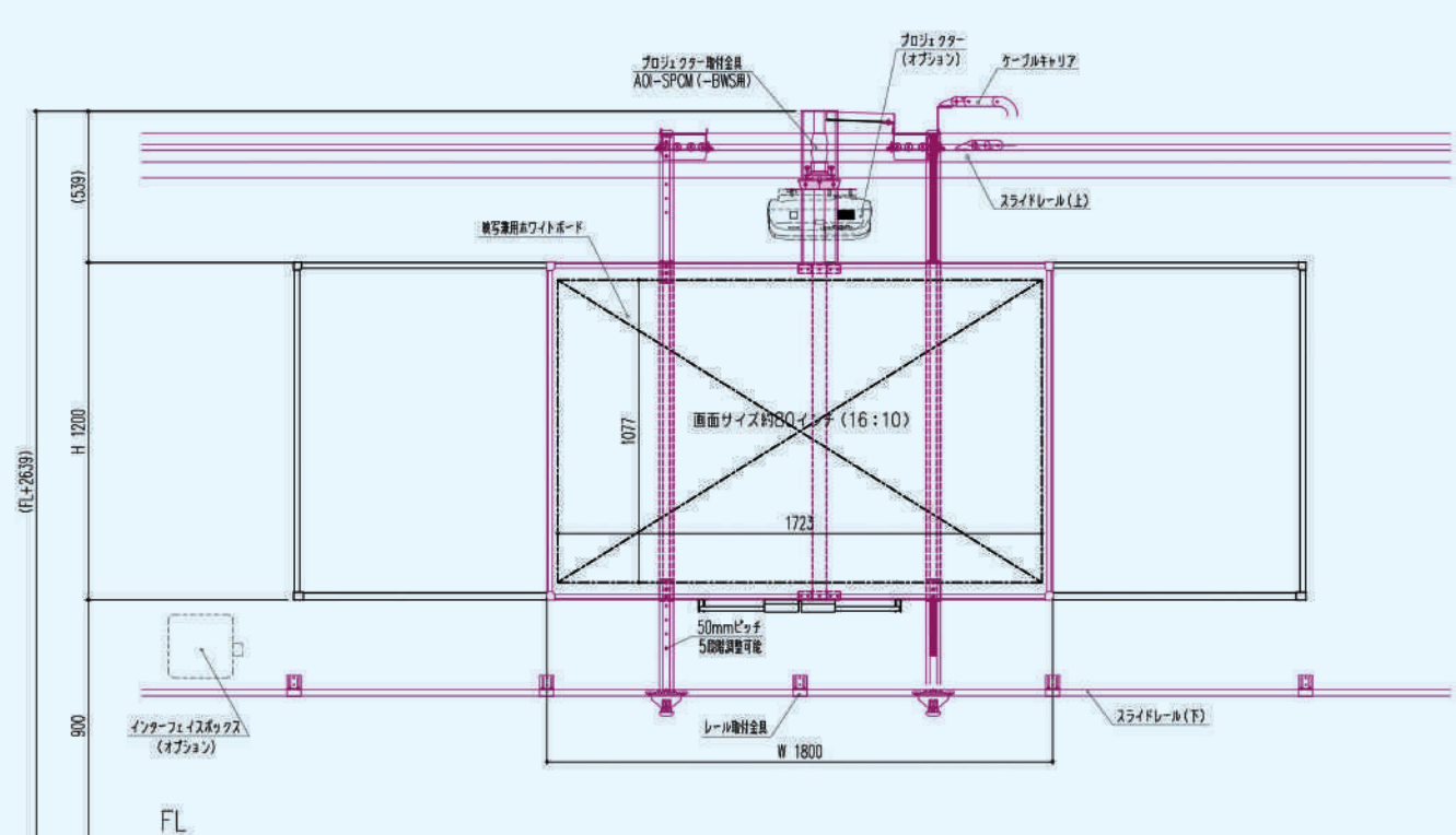
展開図
