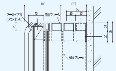
アールピア枠(ソフトエッジ)部 断面図
