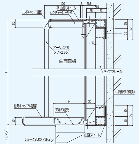
縦断面図
