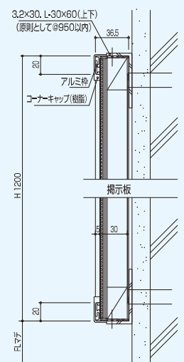
縦断面図
