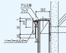
ペーパーホルダー(フック付)の付く場合
