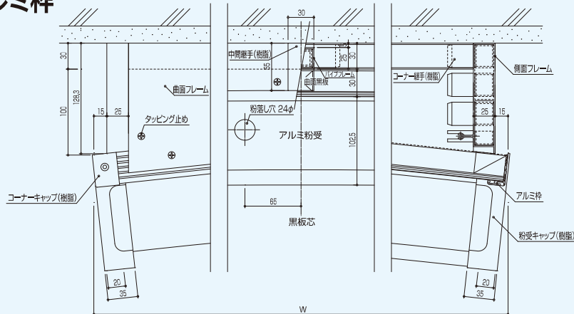
横断面図
