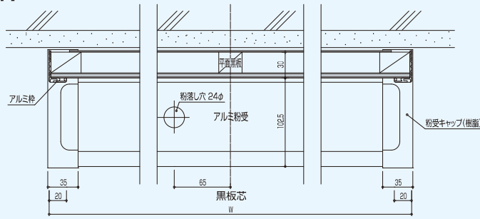
横断面図
