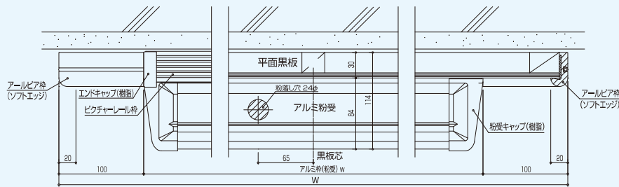
横断面図
