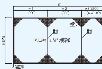
Bパターン:パネル左(右)端基準
