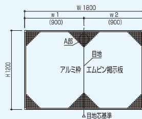
Aパターン:目地芯基準
