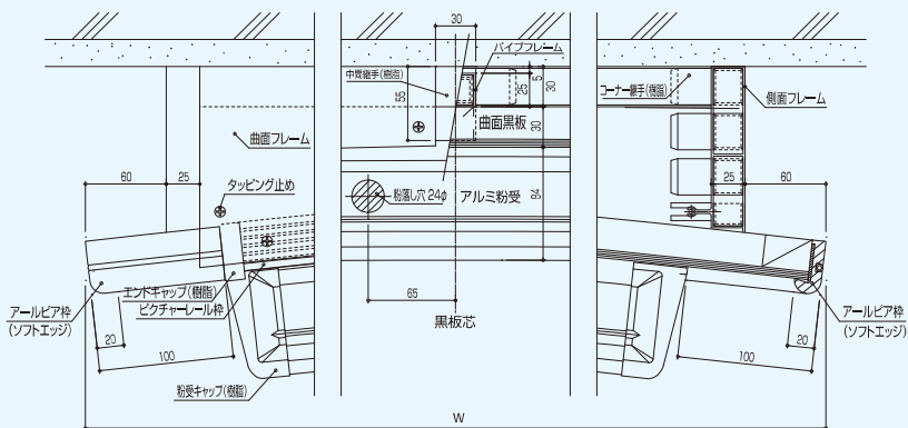
横断面図
