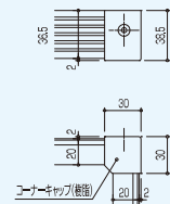
コーナーキャップ 詳細図
