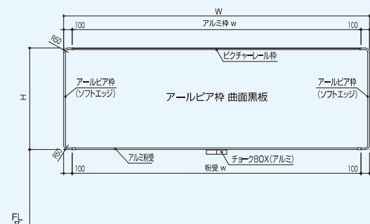
展開図
