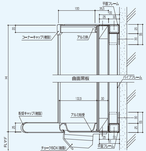
縦断面図
