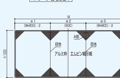
Cパターン:パネル芯基準(目地無視)
