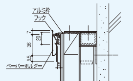
ペーパーホルダー(フック付)の付く場合
