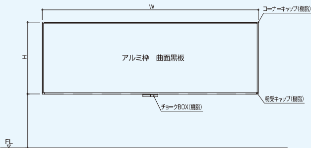
展開図
