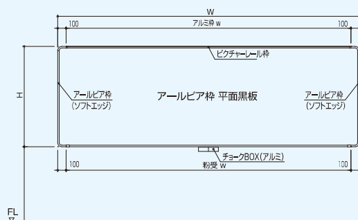
展開図
