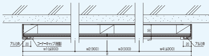
横断面図
