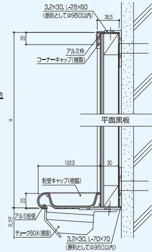
縦断面図
